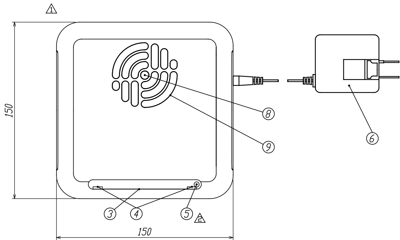
正面図
