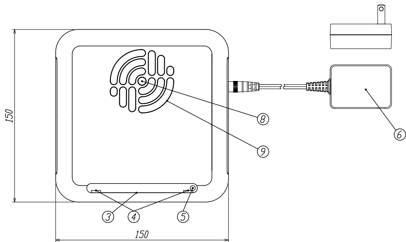
正面図
